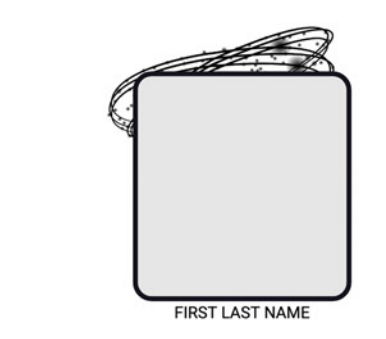
G2S12035
