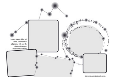
G2S12005
