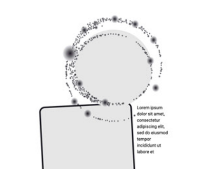
G2S12010
