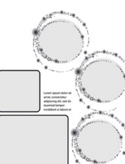
G2S12012
