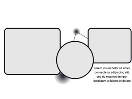
G2S11995
