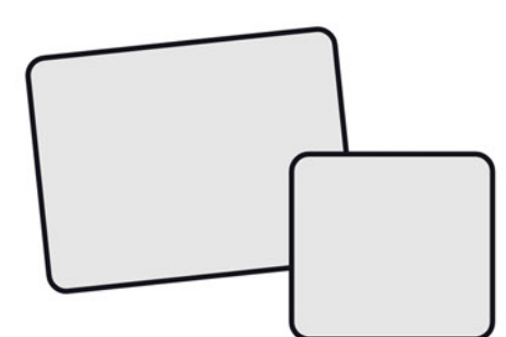
G2S12003
